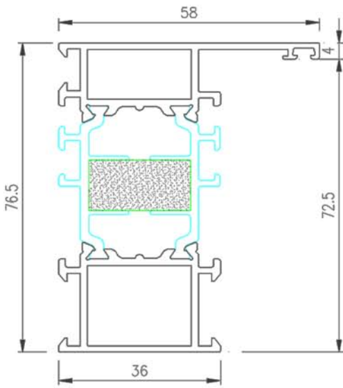
Telaio L (Q)
