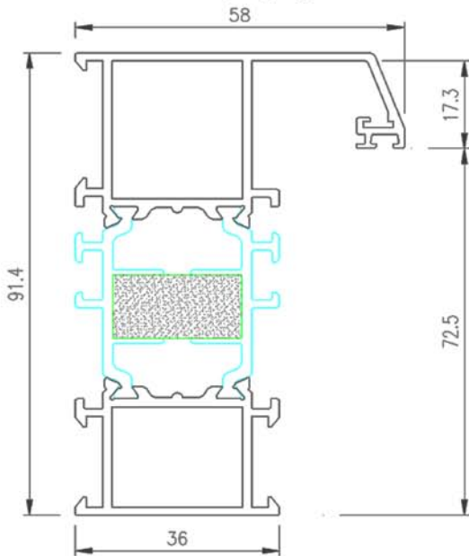
Telaio L (M)
